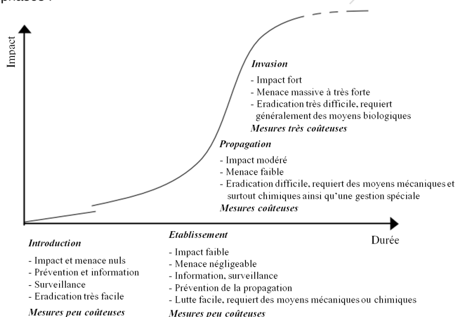
Illustration 1-1 Les quatre phases de la dynamique d'invasion ; exemple des plantes exotiques (tiré de Gigon & Weber 2005) 6
