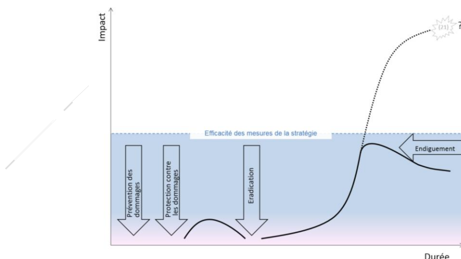
Illustration 1-3 Options d'action durant une invasion biologique pour empêcher la réalisation d'événements tels que ceux mis en évidence dans le scénario de l'OFPP basé sur une dissémination massive d'espèces exotiques envahissantes 21 .
