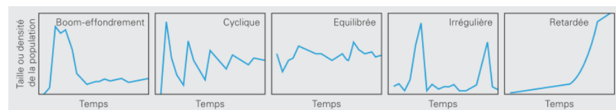
Illustration 1-2 Cinq scénarios possibles d'évolution à long terme pour la moule zébrée et d'autres espèces exotiques (tiré de Kopp & Klappert 2010) 16
